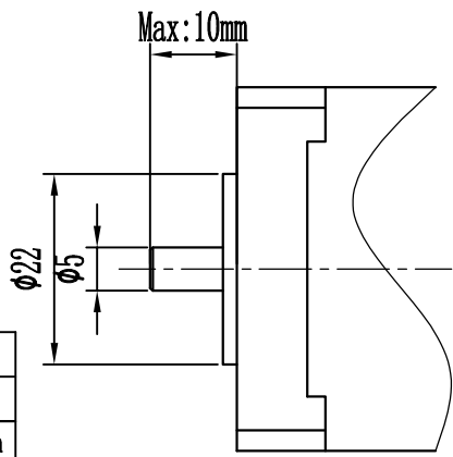
电机配合尺寸示意图 Motor size
